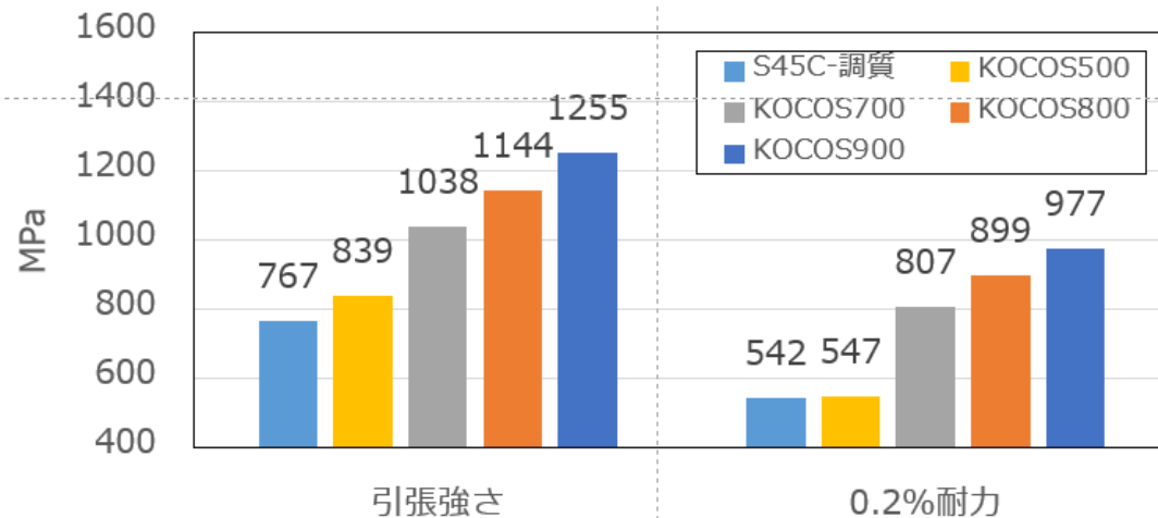
図 KOCOSシリーズ強度比較
