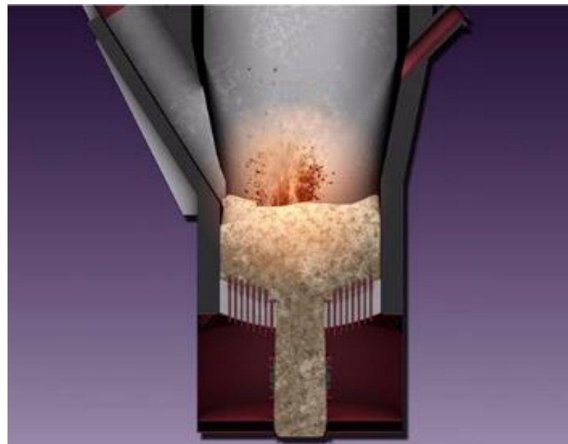
流動層に空気を吹き込む様子
